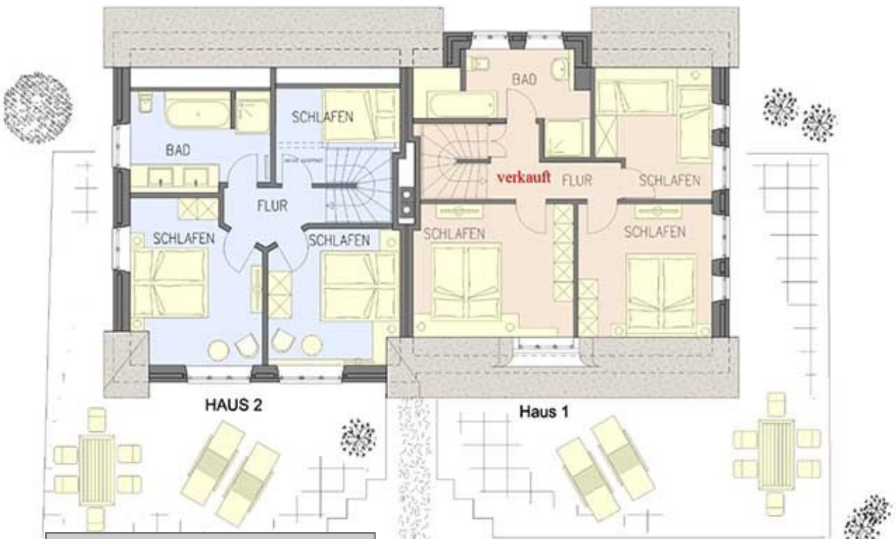
Grundriss Dachgeschoss
