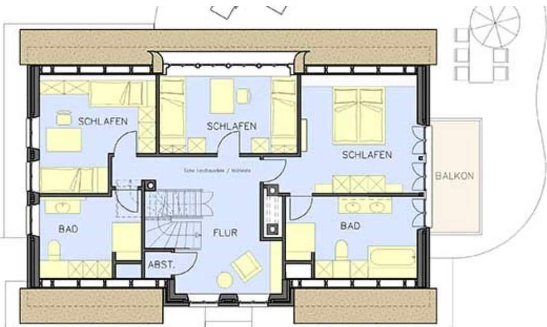
Grundriss Dachgeschoss
