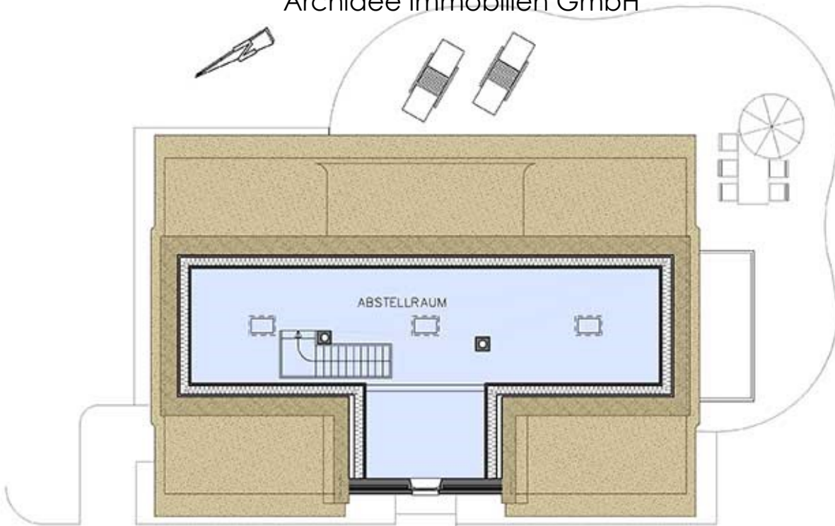
Grundriss Spitzboden
